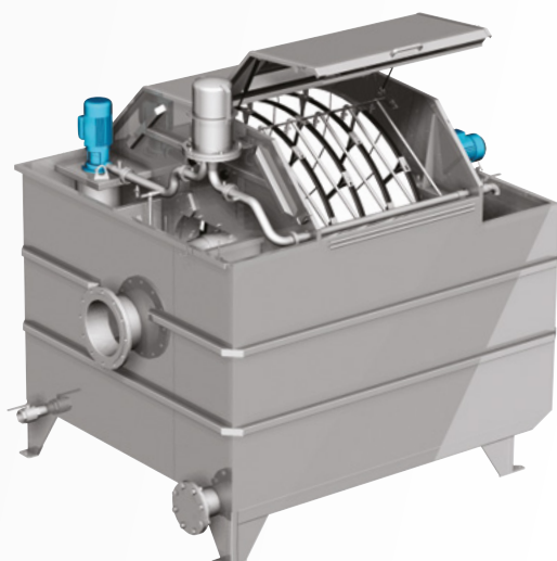
NEREZOVÁ VANA FD_O a FDG_O
